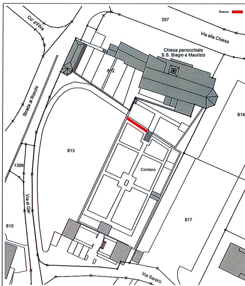
Figura 1: Planimetria progetto loculi
